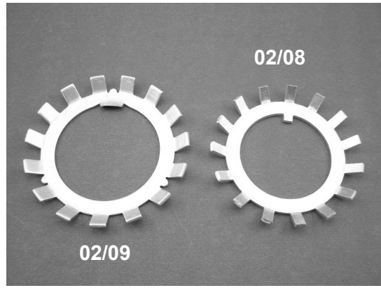
02/08 Araña Hummer ( 35.5m int.) 02/09 Araña Unvan ( 40mm int.)
