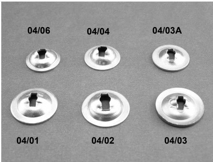
04/01 Cazuela p/clavo Std. 1,2,3,4,5. 04/02 Cazuela p/clavo VW 0 y 00. 04/03 Cazuela p/clavo Datsun. 04/03A Cazuela p/clavo Tsuru. 04/04 Cazuela p/clavo Caribe Corsar. 04/05 Cazuela Guía Chevrolet. 04/06 Cazuela p/clavo Chevy. 04/07 Cazuela de seguridad.
